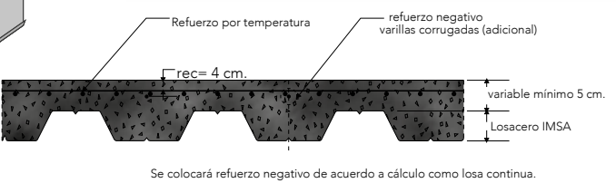
SECCION A-A
